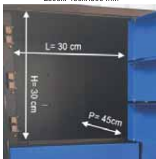
Raggruppamento a 3 scomparti L300xP450xH300 mm
