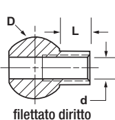
filettato diritto
